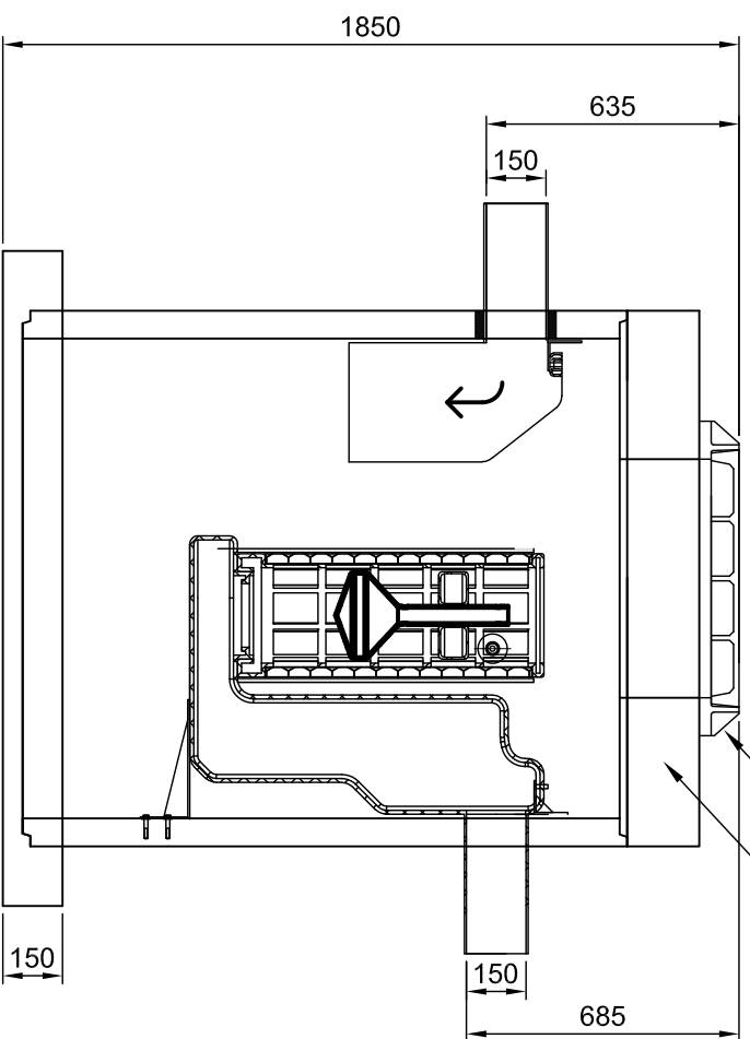
Elevation
